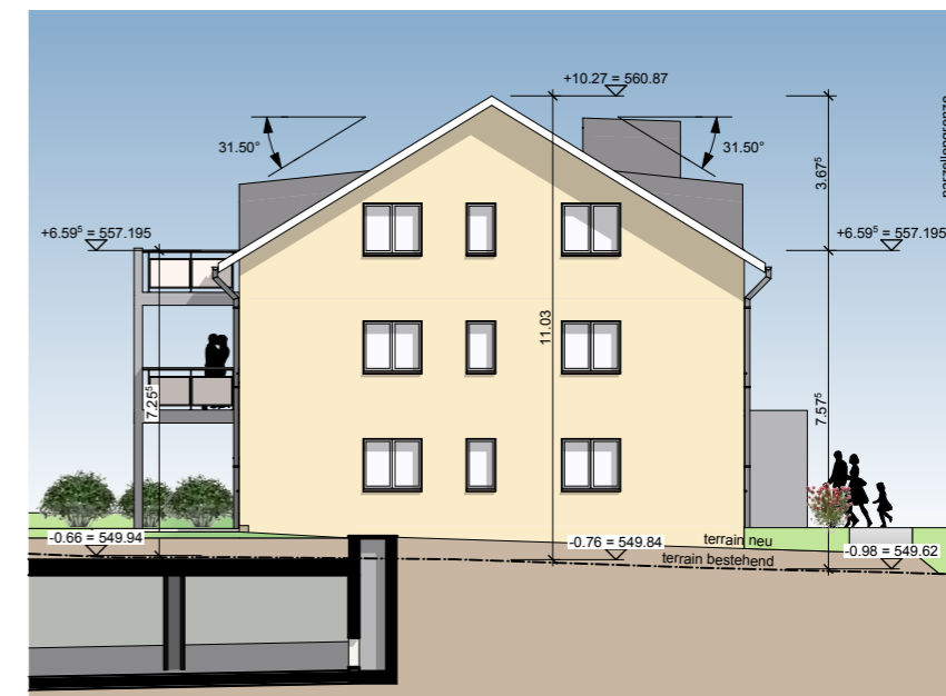
ansicht ost
