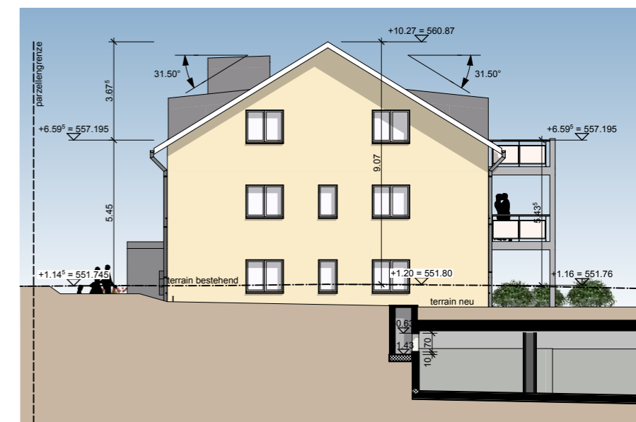
ansicht west
