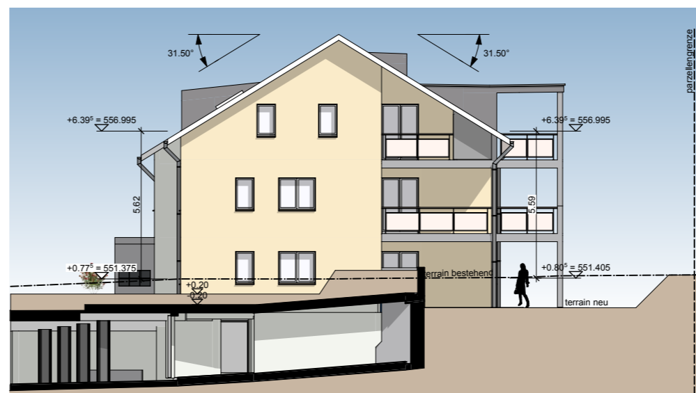
ansicht west
