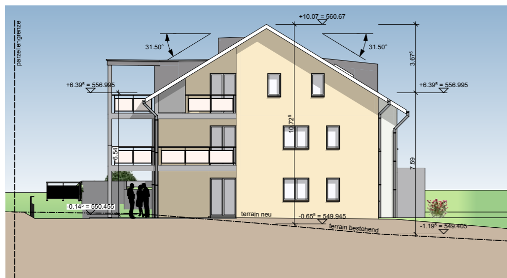
ansicht ost
